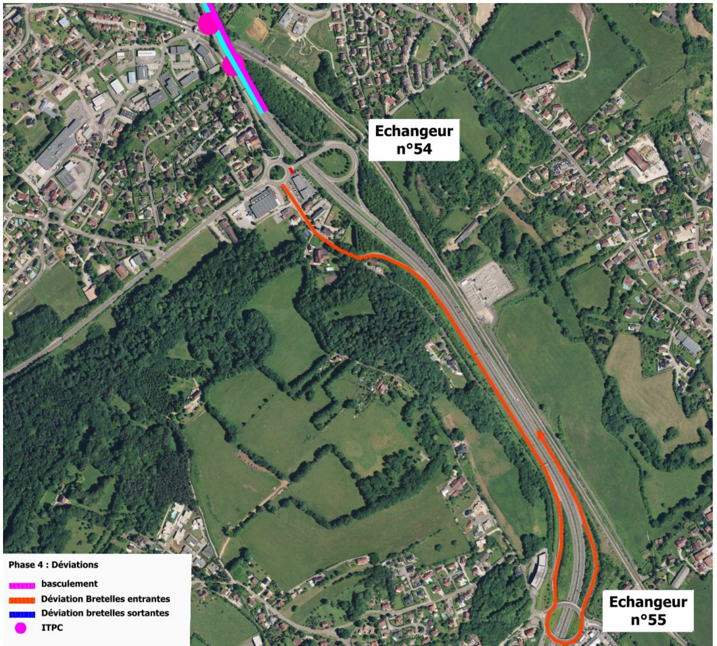
Figure 4: Plan des déviations durant la phase 4 du 9 au 13/08/2021 (la nuit)
